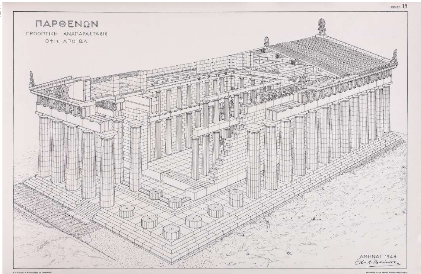
Προοπτική αναπαράσταση του Παρθενώνα. Σχέδιο Α. Ορλάνδου.
