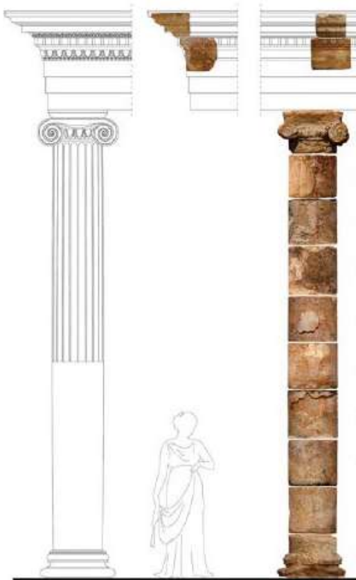
Μαχαιρούς. Ψηφιακή ανακατασκευή (αριστερά) του θριγκού και ενός πλήρους ιωνικού κίονα της περίστυλης εσωτερικής αυλής του βασιλικού λουτροῦ, βάσει της οποίας έγινε η αναστήλωση των κίωνων στον αρχαιολογικό χώρο (δεξιά) (φωτ.: Gyöző Vörös).
