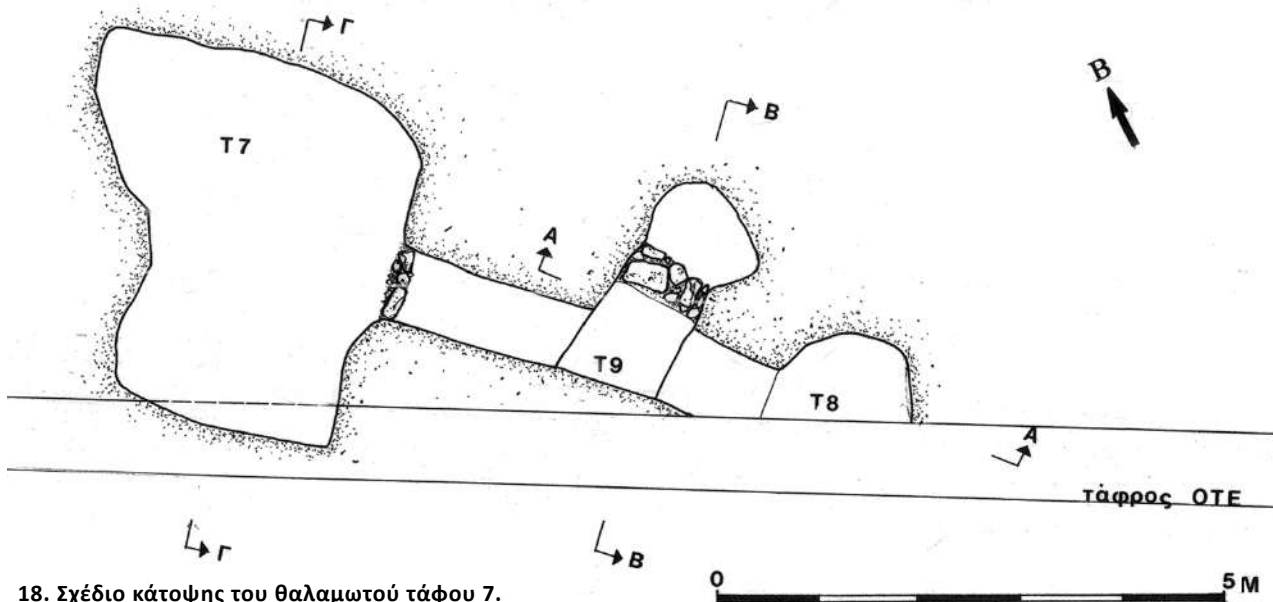
18. Σχέδιο κάτοψης του θαλαμωτού τάφου 7.
