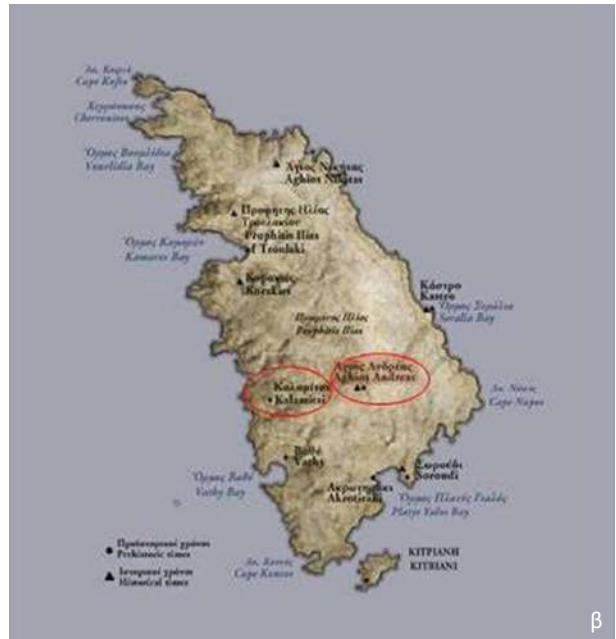
3. α. Χάρτης του Αιγαίου, β. Χάρτης της Σίφνου με τις σημαντικότερες αρχαιολογικές θέσεις.
